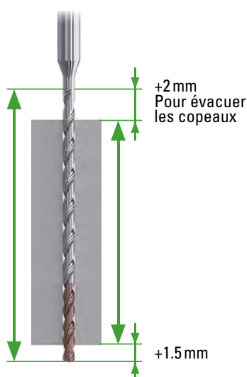
-1- Trous traversants Pièce épaisseur 20 mm
