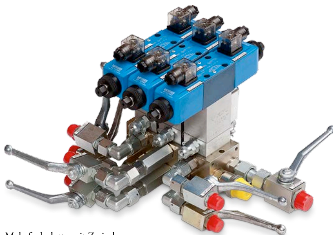
Mehrfachplatte mit Zwischen- platten- und Aufbauventilen. Multistation manifold with sandwiches and directional valves.
