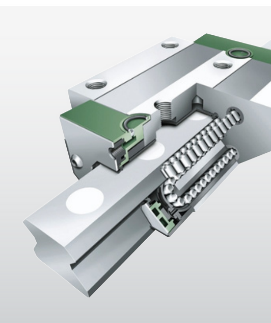
Linearführungen Technique linéaire
